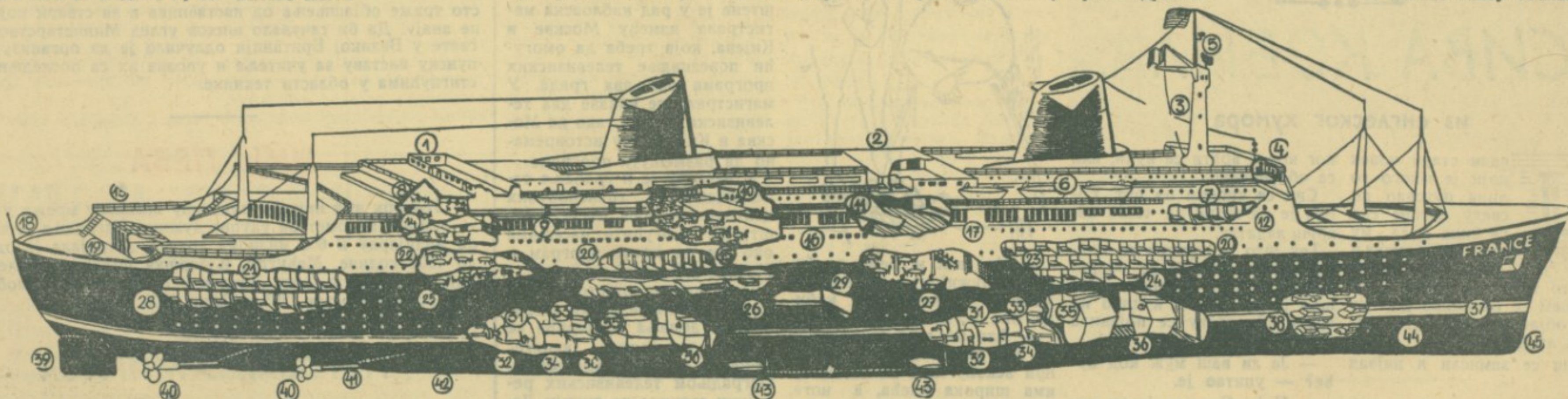
ГОРЊА ПАЛУБА: 1) ЛУНА-ПАРК; 2) ЛУКСУЗНЕ КАБИНЕ У МОЗАИКУ; 3) РАДАРСКА КАТАРКА; 4) НАВИГАТОРСКИ МОСТ; 5) РАДАРСКА АНТЕНА; — МОСТ ЗА ЧАМЦЕ; 6) ЧАМЦИ ЗА 153 ЛИЦА; 7) ОФИЦИРСКЕ КАБИНЕ; — ГОРЊИ МОСТ ЗА ШЕТЊУ; 8) САЛА ЗА ПУШЕЊЕ ПРВЕ КЛАСЕ; 9) ЗАСТАКЉЕНО ШЕТАЛИШТЕ ПРВЕ КЛАСЕ; 10) ВАЛСКА САЛА ПРВЕ КЛАСЕ; 11) НАЈЛЕПША САЛА ЗА ПРЕТСТАВЕ НА ЈЕДНОМ ПЛОВНОМ ОБЈЕКТУ, КОНСТРУИСАНА НА ДВА МОСТА ПОВЕЗАНА СА МЕЗАНИНОМ; 12) ГОРЊЕ ТУРИСТИЧКЕ КАБИНЕ; — ШЕТНИ МОСТ; 13) НЕПОКРИВЕНИ ВАЗЕН ЗА КУПАЊЕ; 14) ВАЛСКА САЛА ТУРИСТИЧКЕ КЛАСЕ; 15) САЛА ЗА ПУШЕЊЕ ТУРИСТИЧКЕ КЛАСЕ; 16) ЗАСТАКЉЕНО ШЕТАЛИШТЕ ТУРИСТИЧКЕ КЛАСЕ; 17) КОНЦЕРТНА САЛА; — ГОРЊИ МОСТ; 18) ЗАДЊА ПЛАЖА ТУРИСТИЧКЕ КЛАСЕ; 19) ТУРИСТИЧКИ ВАЗЕН ЗА ПЛИВАЊЕ; 20) КАБИНЕ ПРВЕ КЛАСЕ; — ГЛАВНИ МОСТ; 21) КАБИНА ТУРИСТИЧКЕ КЛАСЕ; 22) ГОРЊА ТРПЕЗАРИЈА ТУРИСТИЧКЕ КЛАСЕ; 23) ЗАЈЕДНИЧКЕ К. ВИНЕ; — МОСТ А; 24) КАБИНЕ ТУРИСТИЧКЕ КЛАСЕ; 25) ТРПЕЗАРИЈА ТУРИСТИЧКЕ КЛАСЕ; 26) КУХИЊЕ; 27) ТРПЕЗАРИЈА ПРВЕ КЛАСЕ; 28) КАБИНЕ ТУРИСТИЧКЕ КЛАСЕ; — МОСТ Д; 29) ВАЗЕН ПРВЕ КЛАСЕ; — ОДЕЉЕЊА ЗА МАШИНЕ; 30) МЕСТО РАЧВАЊА ЕЛИСА; 31) РЕГУЛАТОР ЗА БРЗИНУ; 32) ТУРБИНА НР; 33) ТУРБИНА МР; 34) ГЛАВНИ КОНДЕНЗАТОР; 35) КАЗАН ЗА ПРЕЧИШЋАВАЊЕ МОРСKE ВОДЕ; — ОДЕЉЕЊЕ ЗА ЗАГРЕВАЊЕ; 36) КОТЛОВИ; 37) ЛИНИЈА ГАЗА; 38) ГАРАЖА; 39) КРМА; 40) ЕЛИСА; 41) ДРЖАЧ ЕЛИСЕ; 42) КРИЛНИ ПРЕНОСНИК; 43) СТАБИЛИЗАТОР ПРОТИВ ЉУЉАЊА; 44) ВОК; 45) КЉУН БРОДА
