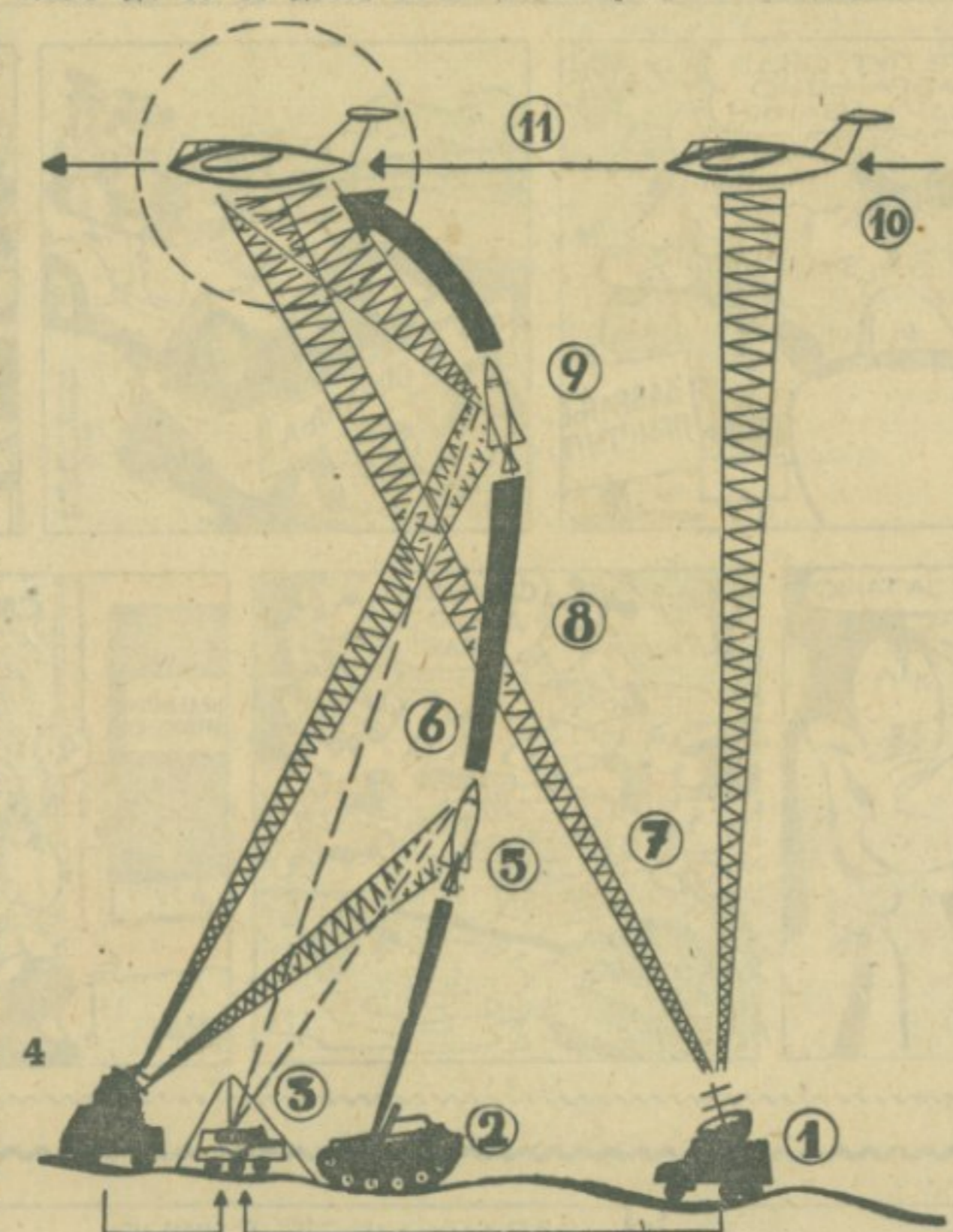
1) РАДИОЛОКАТОР ЗА ПРАВЕЊЕ ЦИЉА; 2) УРЕЂАЈ ЗА ИСПАЉИВАЊЕ РАКЕТА; 3) УРЕЂАЈ ЗА ПРИМАЊЕ ПОДАТАКА ОД РАДИОЛОКАТОРА И УПРАВЉАЊЕ РАКЕТОМ; 4) РАДИОЛОКАТОР ЗА ПРАВЕЊЕ РАКЕТЕ; 5) ПОТИВАВИОНСКА РАКЕТА; 6) ЗАПОВЕСТИ ЗА ИСПРАВКЕ РАДИОСТАНИЦЕ; 7) ТАЛАСИ РАДИОЛОКАТОРА; 8) ПУТ РАКЕТЕ; 9) НА ОДРЕЂЕНОЈ УДАЉЕНОСТИ ПОЧИЊЕ ДЕЛОВАТИ УРЕЂАЈ ЗА САМОСТАЈНО УПРАВЉАЊЕ РАКЕТОМ; 10) ЦИЉ У ВАЗДУХУ И ПРАВАЦ ЊЕГОВОГ КРЕТАЊА; 11) ОКРУГ УДАЉЕНОСТИ У КОЈЕ РАКЕТА АУТОМАТСКИ ЕКСПЛОДИРА.
