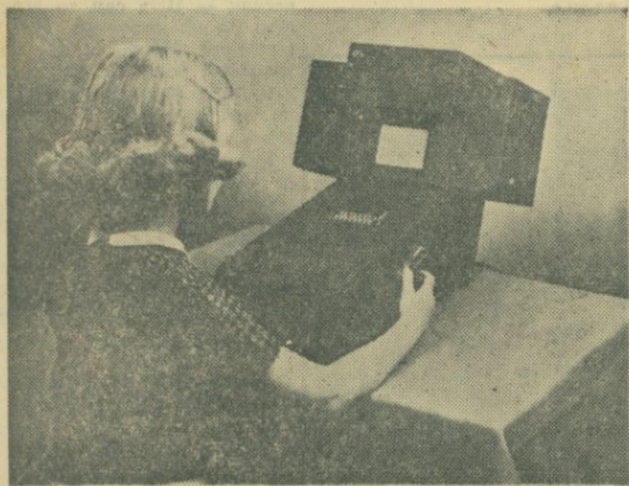
ЈЕДАН ОД КОМПЛИКОВАНИЈИХ МОДЕЛА СКИНЕРОВЕ МАШИНЕ ЗА УЧЕЊЕ КОЈА ПОСТАВЉА ПИТАЊА ИЗ АРИТМЕТИКЕ. ВАК МОЖЕ ДА ТРАЖИ ДРУГИ ПРОБЛЕМ САМО АКО ЈЕ ПРЕТХОДНИ ОДГОВОР ТАЧАН
