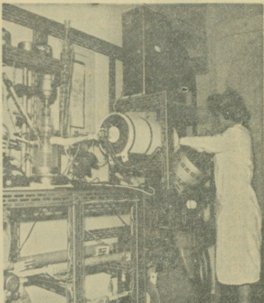
ПЕЋ ЗА СИНТЕРОВАЊЕ УРАНИЈУМ ДИОКСИДА
