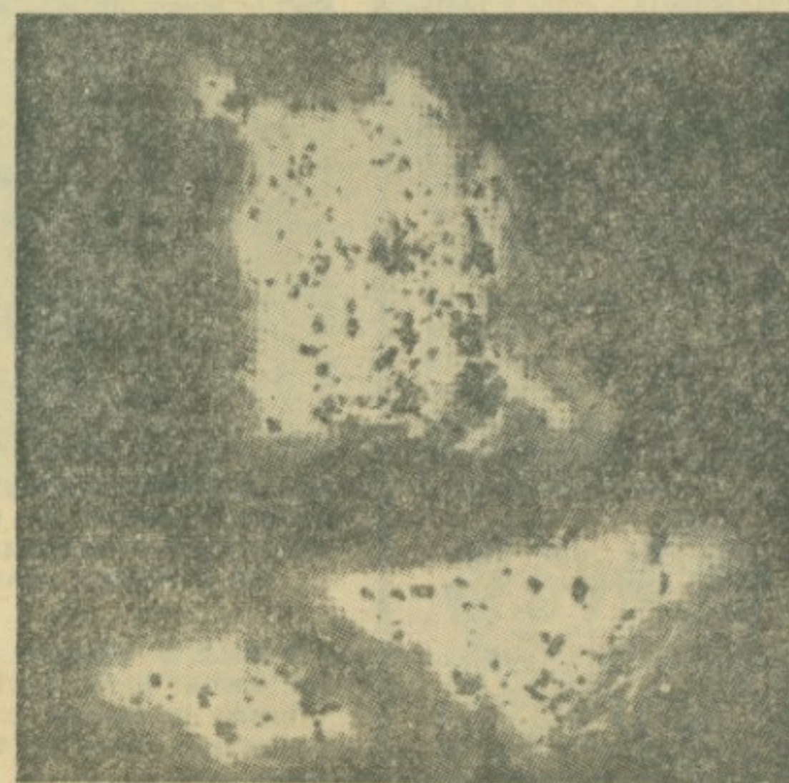
ПРАХ УРАНИЈУМ ДИОКСИДА УВЕЛИЧАЊЕМ ВИШЕ ХИЉАДА ПУТА ПОДСЕЋА НА НАЈМОДЕРНИЈЕ КЕРАМИЧКЕ СКУЛПТУРЕ
