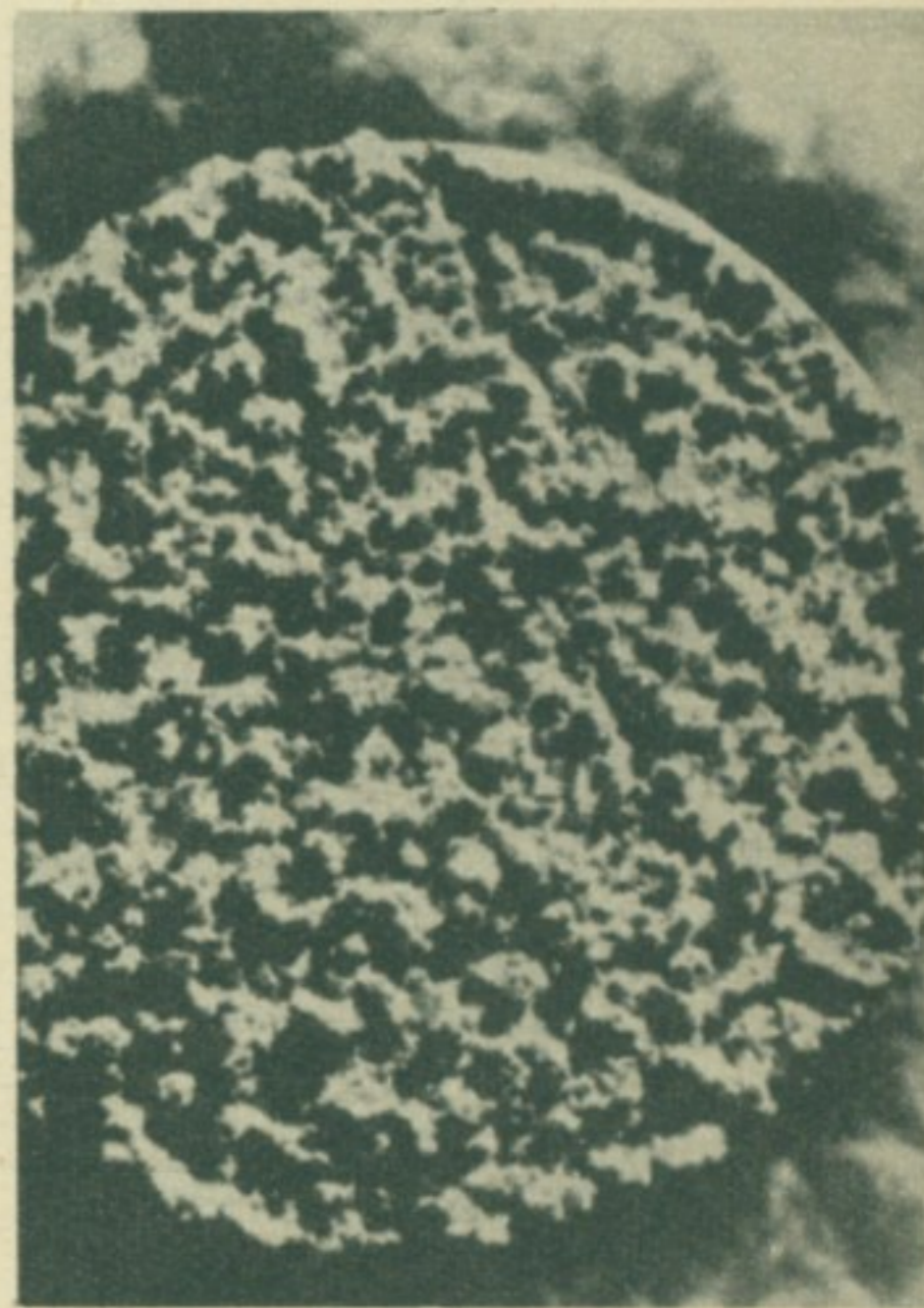
Комад алуминијума је потпуно деформисан пошто је један минут издржао кишу јачине 1476 км/час.
