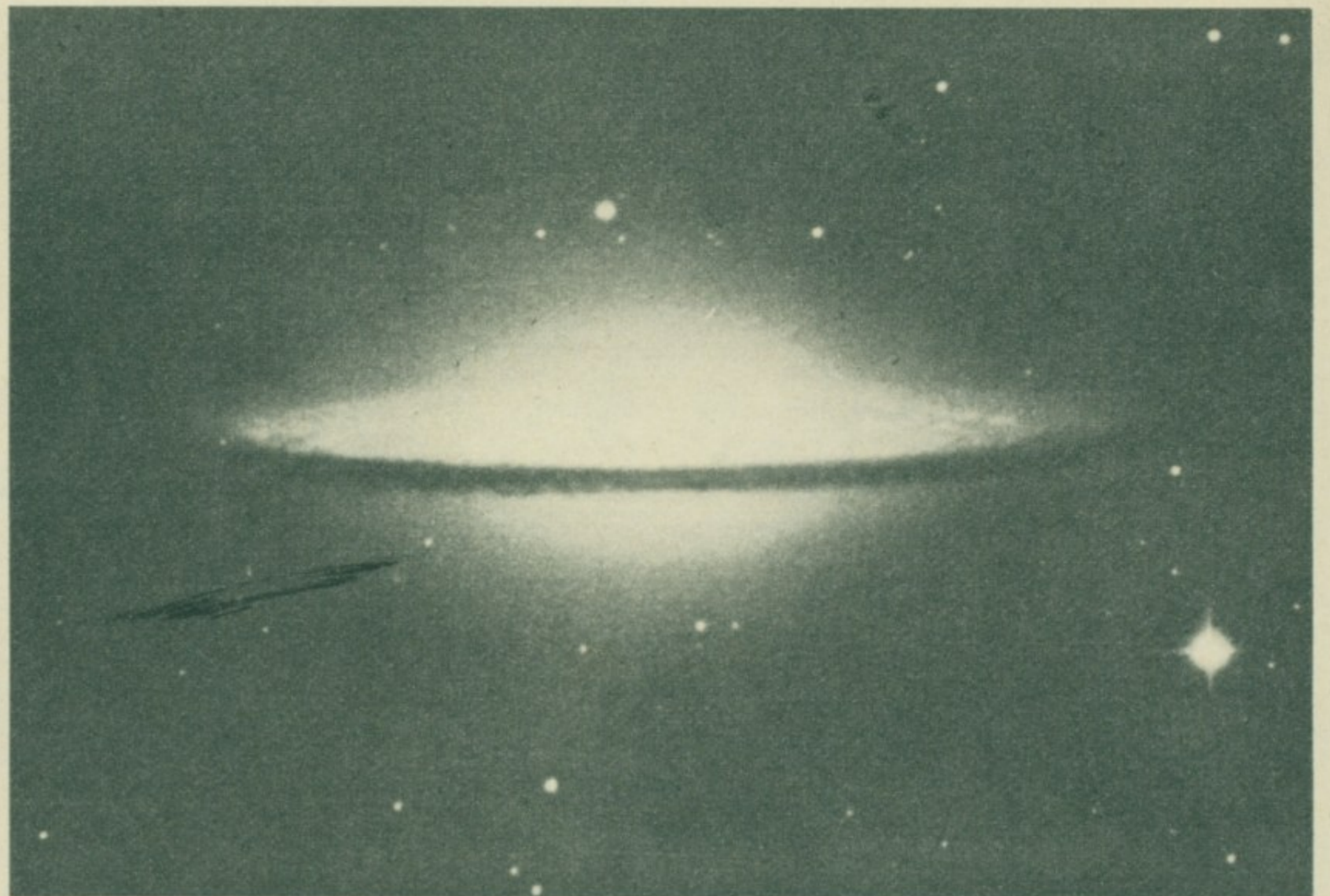
ГАЛАКСИЈА САЗВЕЖЂА ДЕВИЦЕ. МАТЕРИЈА ЗГУСНУТА ТАКО ДА ЧИНИ КРУГ ПОТПУНО ЗАКЛАЊА СРЕДИШНЕ ЗВЕЗДЕ. СНИМАК ОПСЕРВАТОРИЈЕ ПАЛОМАР.
