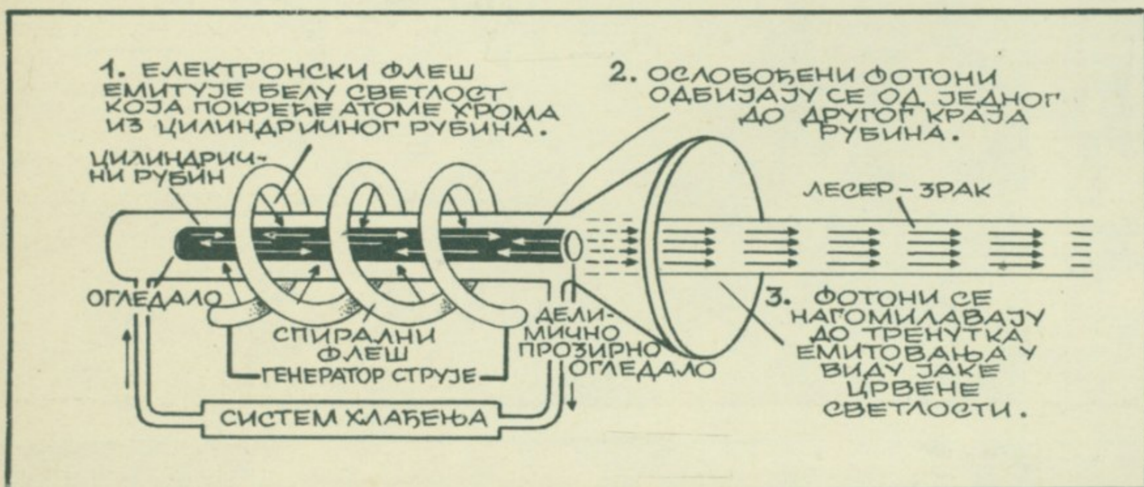
ЛАСЕР СА СИНТЕТИЧКИМ РУБИНОМ. ШЕМА ПРИКАЗУЈЕ ЊЕГОВ РАД У ГЛАВНИМ ФАЗАМА: ФЛЕШ ЕМИТУЈЕ БЕЛУ СВЕТЛОСТ КОЈА ПОКРЕЋЕ АТОМЕ ХРОМА; ОДБИЈАЊЕ ФОТОНА ОД ЈЕДНОГ ДО ДРУГОГ КРАЈА РУБИНА; ЕМИТОВАЊЕ ФОТОНА У ВИДУ ЦРВЕНЕ СВЕТЛОСТИ.
