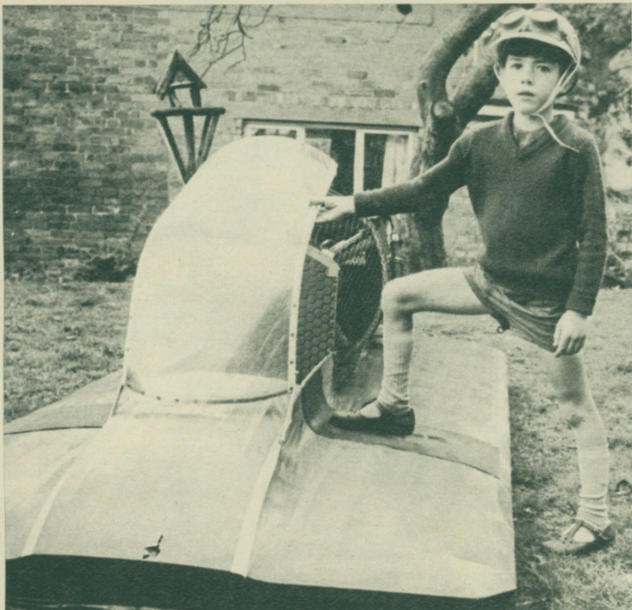
МАЛИ КОНСТРУКТОР. Док се већина његових вршњака вози тротинетом или трициклом, седмогодишњи Гај Мејер из Белтона у Енглеској има сопствени ховеркрафт. Ово возило, које се креће на ваздушним јастуцима, мали конструктор је сам направио искористивши при том један стари мотоцикл. Без обзира на очеву финансијску и стручну помоћ то је велики успех малог Гаја.
