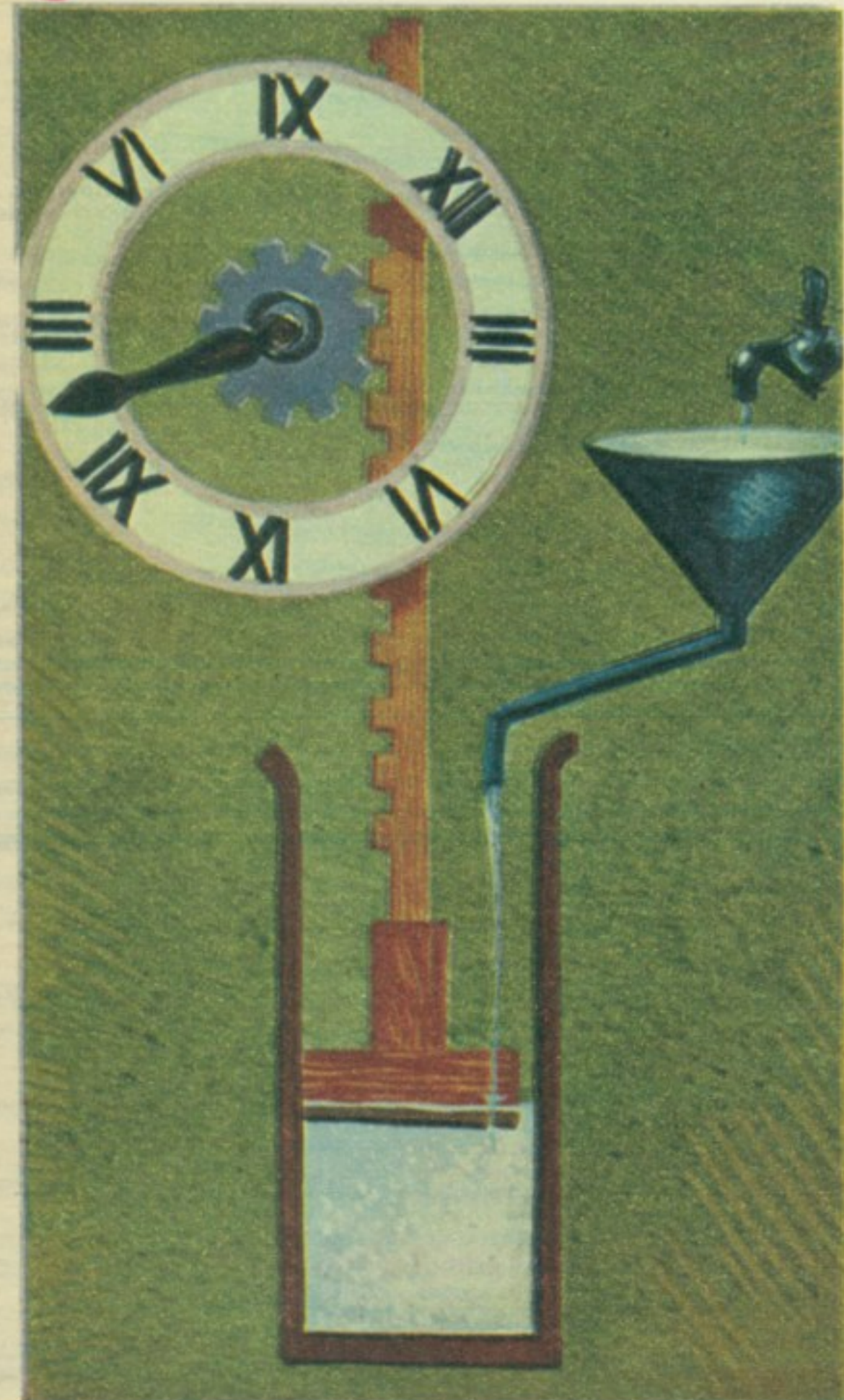
8 ВОДЕНИ САТ — Вода, пунећи посуду уједначеним ритмом, подиже пловећи клип са назубљеном полугом која покреће горњи зупчаник а са њим и казаљку. Употребљавали су га стари Грци и Римљани.
