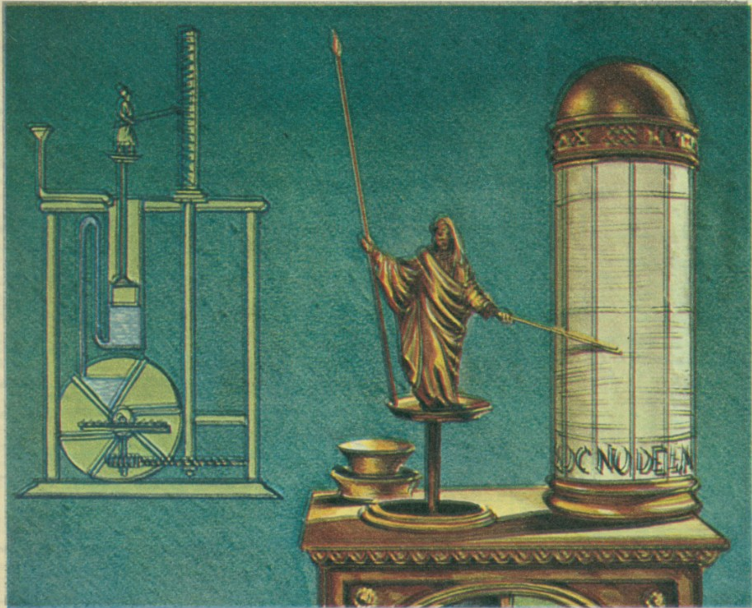
6 ВОДЕНИ САТ — Овај веома леп часовник ради на истом принципу као и претходни а стрела у руци фигурице показује време на скали. У доба чувеног грчког говорника Демостена овакви сатови употребљавали су се у атинским судовима да би ограничили говоре адвоката.
