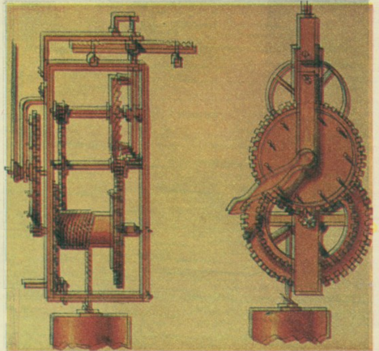
7 МЕХАНИЧКИ ЧАСОВНИК — Ово је шема механичког сата. Цилиндар, који се окреће помоћу тега, покреће казаљку за показивање часова на скали и преко разних зупчаника покреће осу полуге. Тегови регулишу ритам рада часовника.
