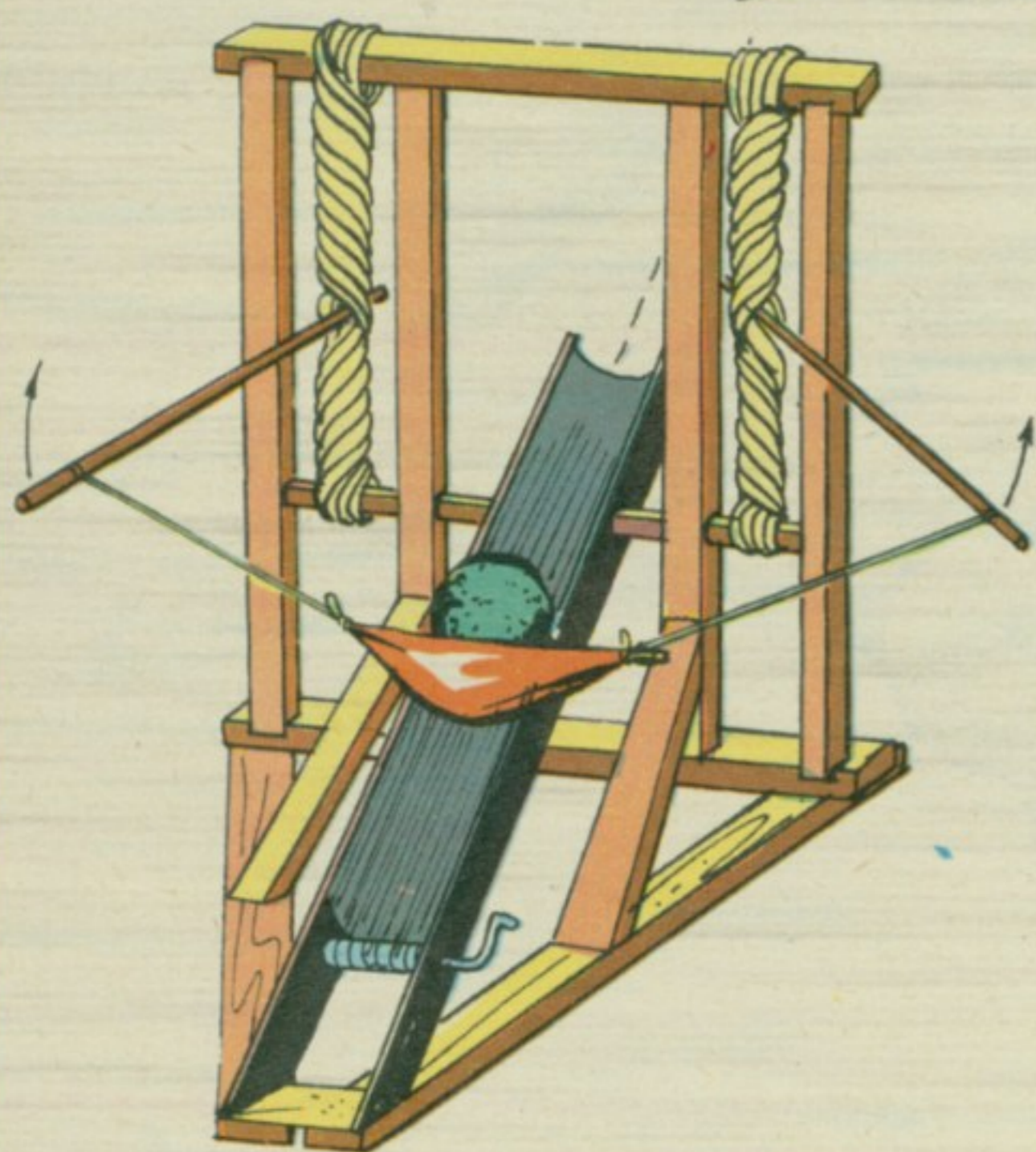
БАЦАЧ КАМЕЊА - ПЕТРОБОЛА
