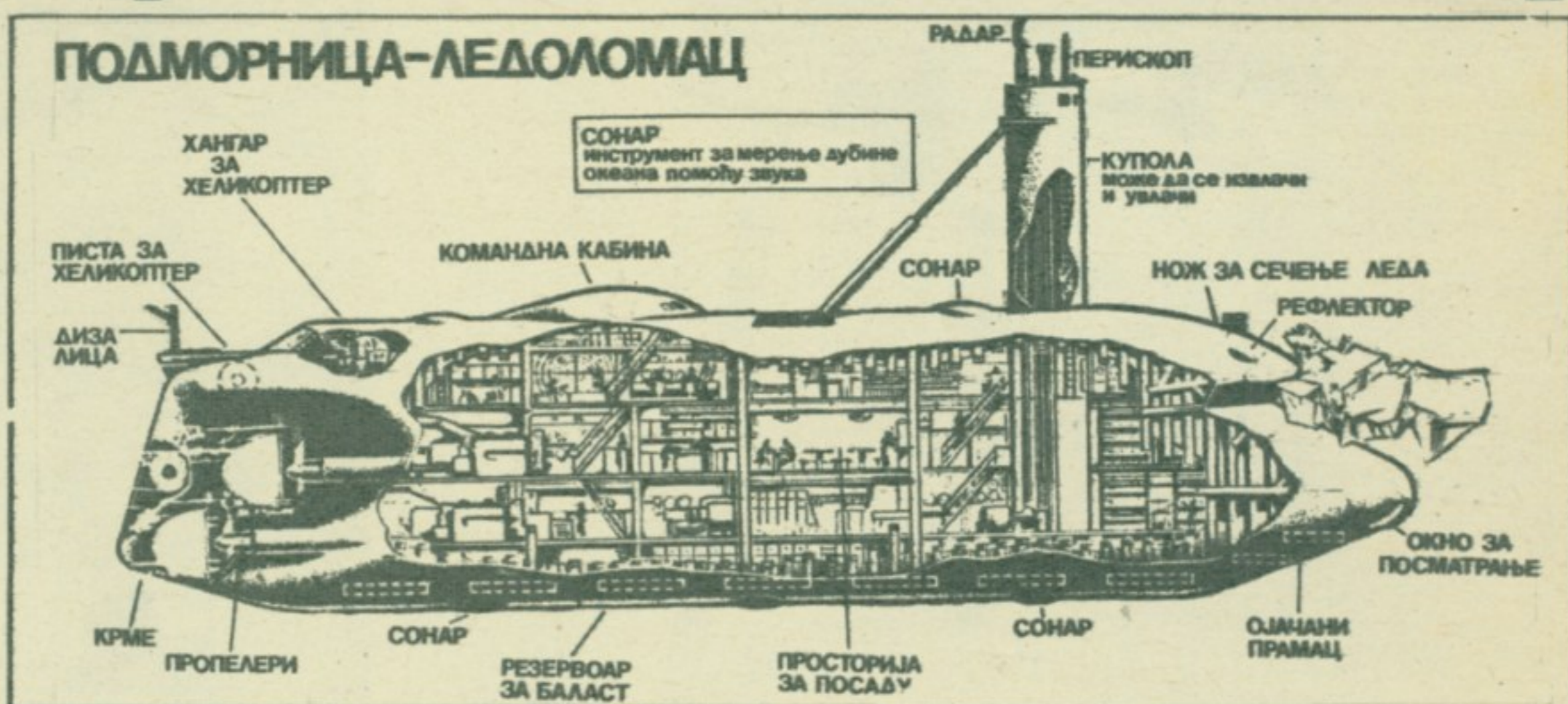
ПРЕСЕК ПОДМОРНИЦЕ-ЛЕДОЛОМЦА НА КОЈОЈ СЕ ВИДЕ РАЗНЕ ПРОСТОРИЈЕ ЗА ЖИВОТ И РАД, КАО И РАЗНИ ВАЖНИЈИ ДЕЛОВИ БРОДА. ВЕЋИ ДЕО ПОДМОРНИЦЕ НАЛАЗИ СЕ ИСПОД ПОВРШИНЕ.
