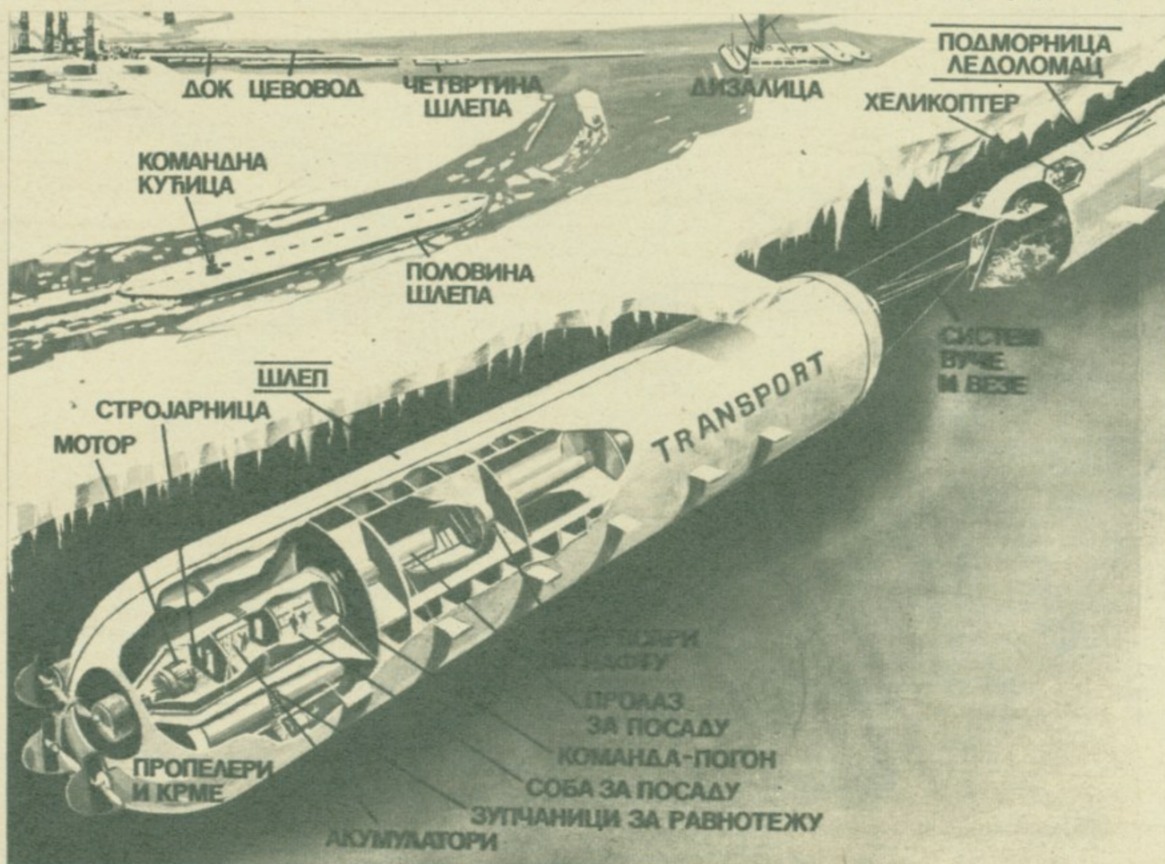
САМО ОВАКАВ ШЛЕП КОГА ВУЧЕ ПОДМОРНИЦА-ЛЕДОЛОМАЦ МОЖЕ БЕЗБЕДНО И БРЗО ДА ПРЕВЕЗЕ ОГРОМАН ТЕРЕТ КРОЗ ОПАСНЕ ВОДЕ СЕВЕРНОГ И ЈУЖНОГ ПОЛА.
