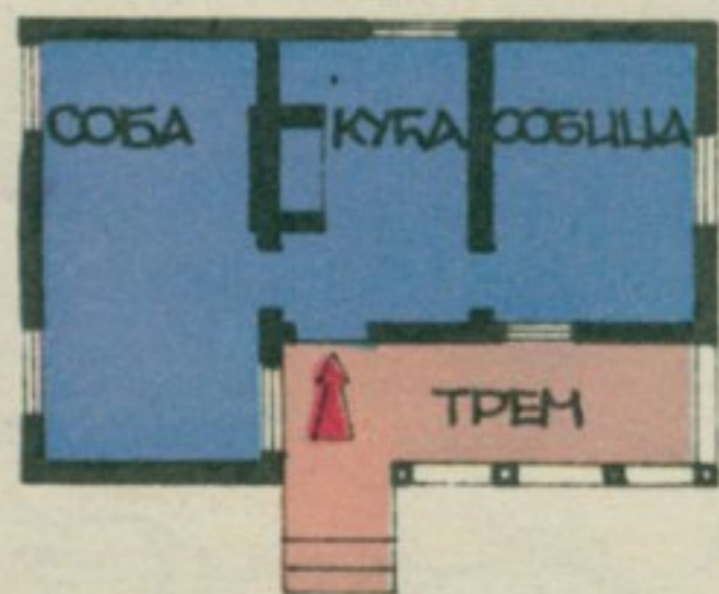
ОСНОВА МОРАВСКЕ КУЋЕ
