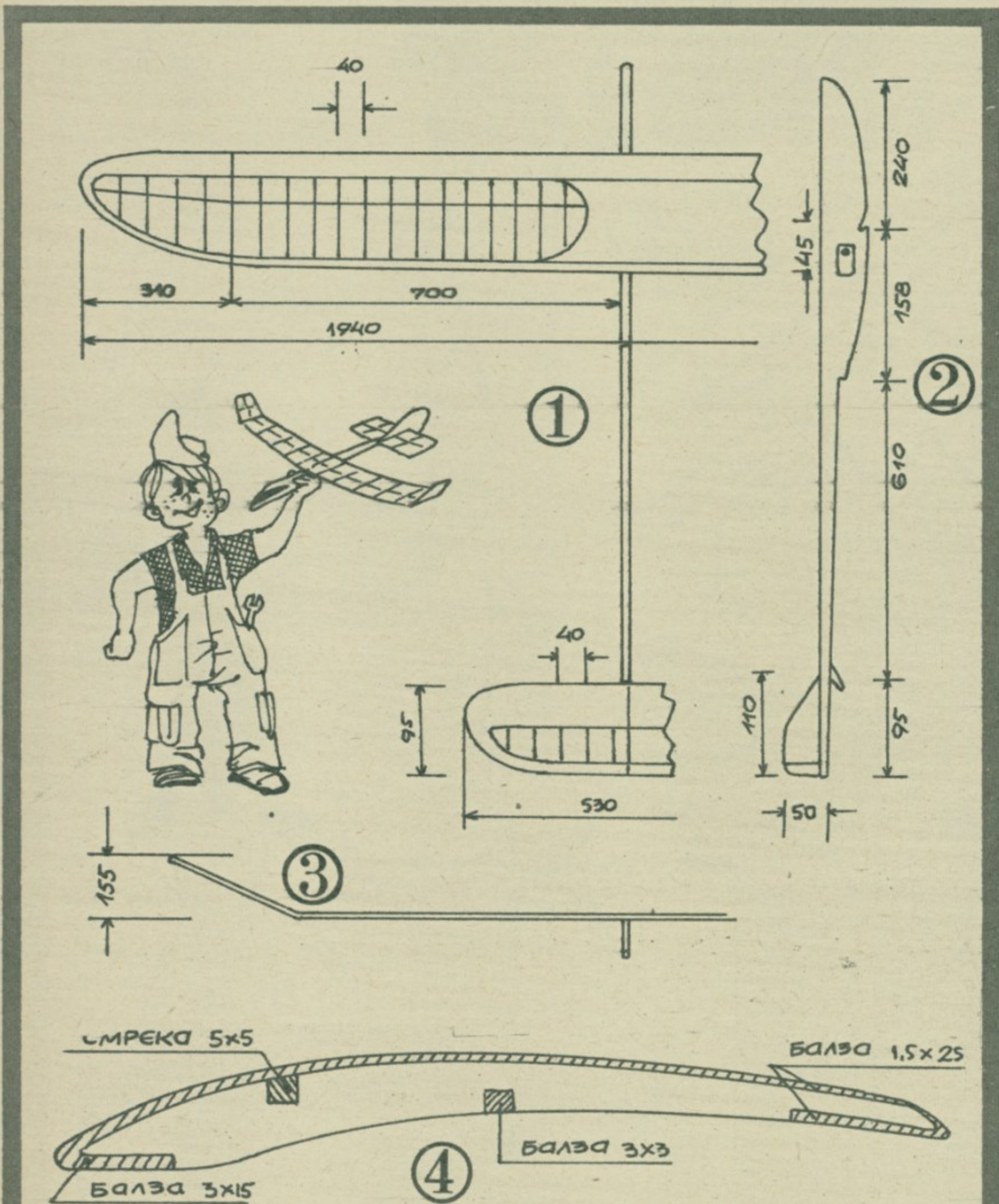
СКИЦА ЈЕДРИЛИЦЕ ЗА СЛОБОДАН ЛЕТ (мере изражене у милиметрима): 1. Изглед модела одозго; 2. Изглед модела са стране; 3. Изглед профила крила; 4. Попречни пресек крила.
