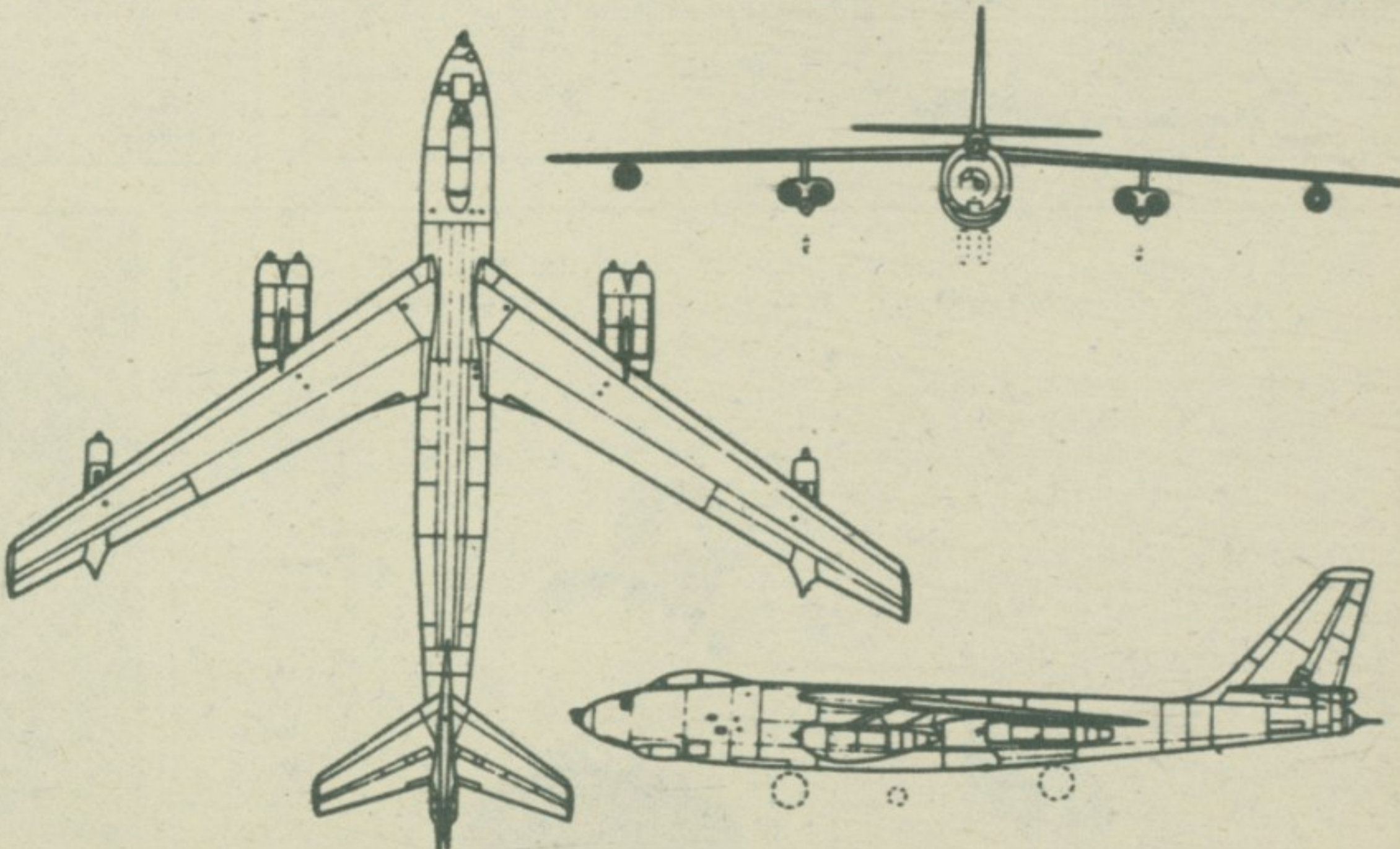
Три цртежа авиона В-47 стратоџет, првог млазног бомбардера са стреластим крилима и шест мотора, посматраног одозго, спреда и бочно.
