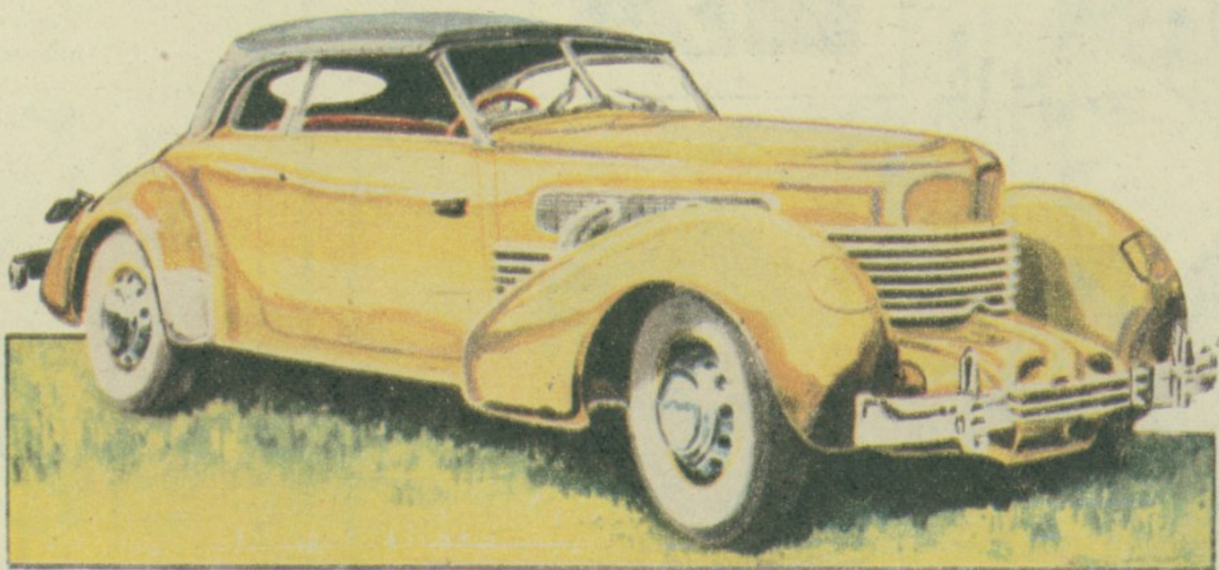
CORD MODELE 812 1937. — Појава „корд“ модела представљала је корак напред у развоју аутомобилизма. Предња вуча и независно вешање на сва четири точка били су гаранција стабилности на путу. Са мотором од 4700 кубика, јачине 120—180 „коња“, постигао брзину до 180 km/h.
