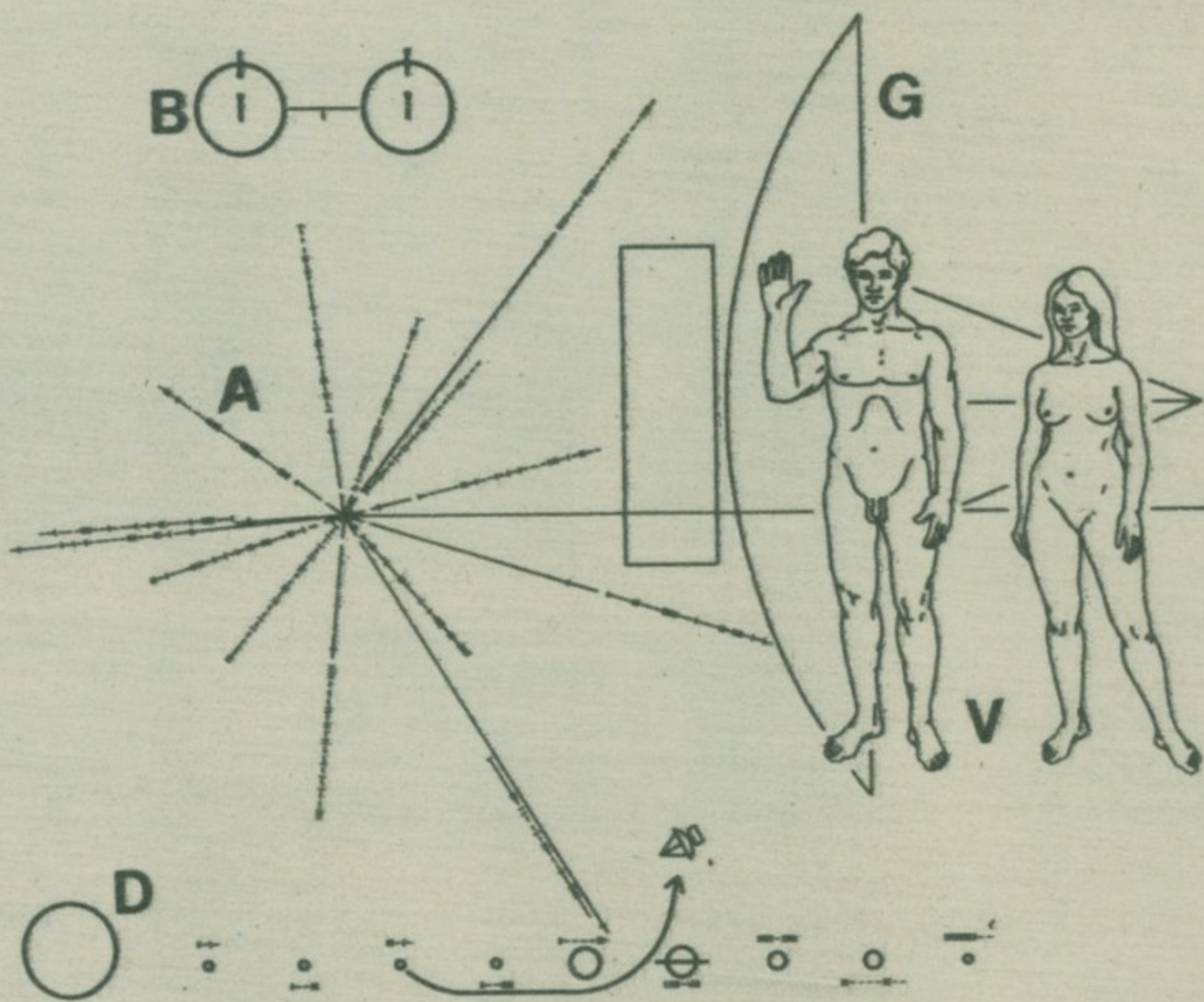
Прва порука Земље васиони: цртеж изгравиран на две плaketе на детелицама „Пионир“.
