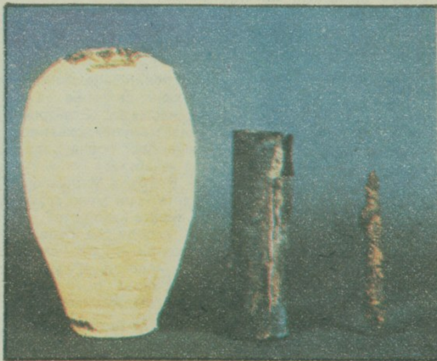
Антички познаваоци електрицитета: делови „багдадске батерије“ изложени у Ирачком музеју.
