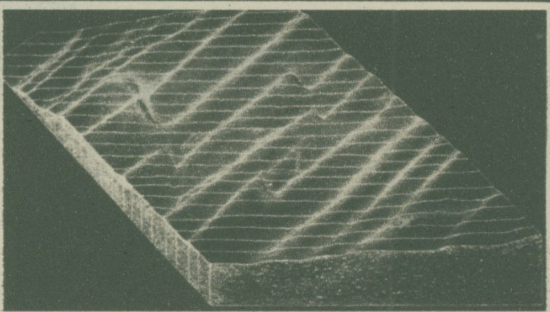
„Снимак“ кристала силицијума: гредасте степенице су висине само колико један атом. Узрслине означавају неправилне везе у кристалу.
