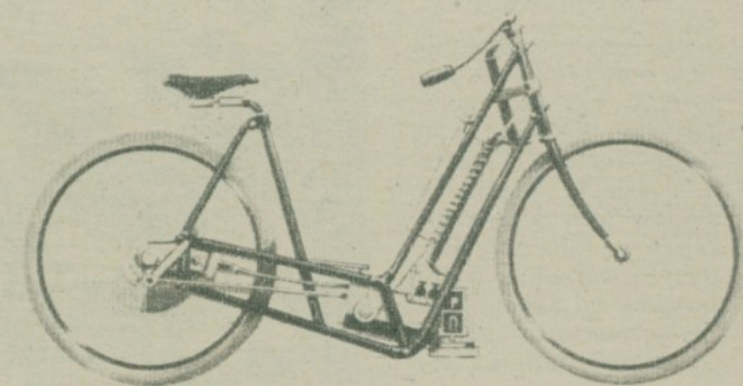
Хилдербрандов и Волфинперов модел представљао је значајан корак.
