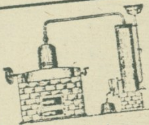
Slika br. 1 pokazuje kazan komplet uzidan najnovijeg tipa sa cilindričadnja-kom, mogu biti sadržine od 80 do 1000 litara, a najpodesniji su od oko 500 litara. Ovakvi se kazani ne pokreću sa svog mesta.
