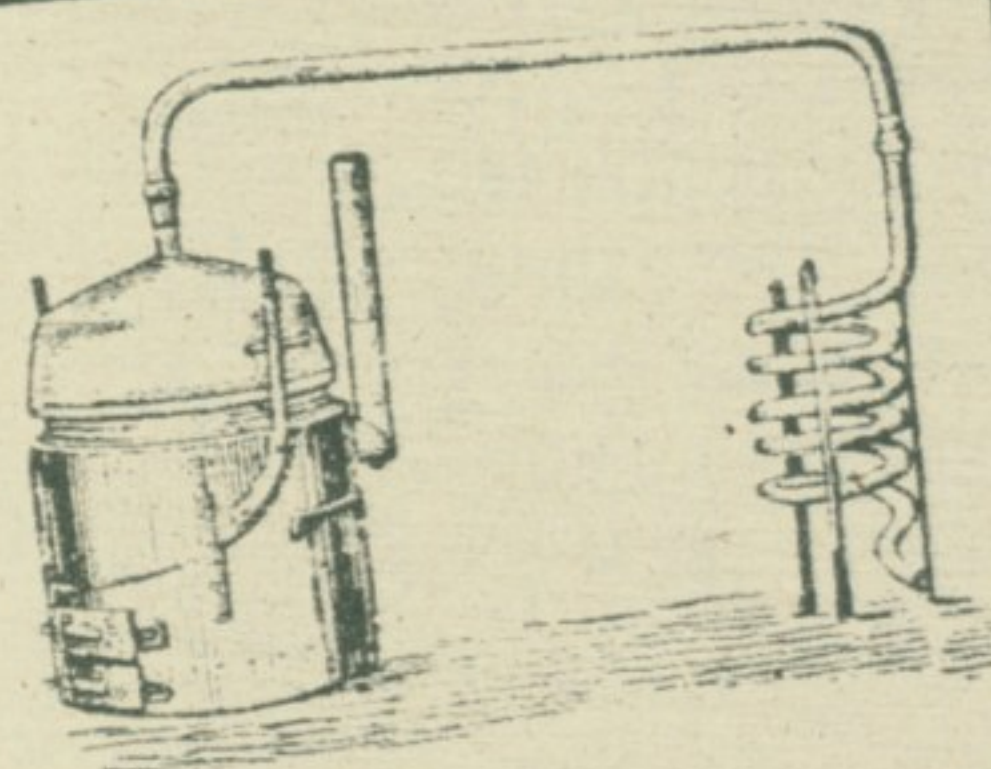
Slika br. 3 kazan komplet sa željeznom peći , koji se ispražnjuje pomoću izvrtanja, kao što pokazuje slika br. 2, veoma podesan za pečenje lozovog koma, a isto za prepećanje rakije.
