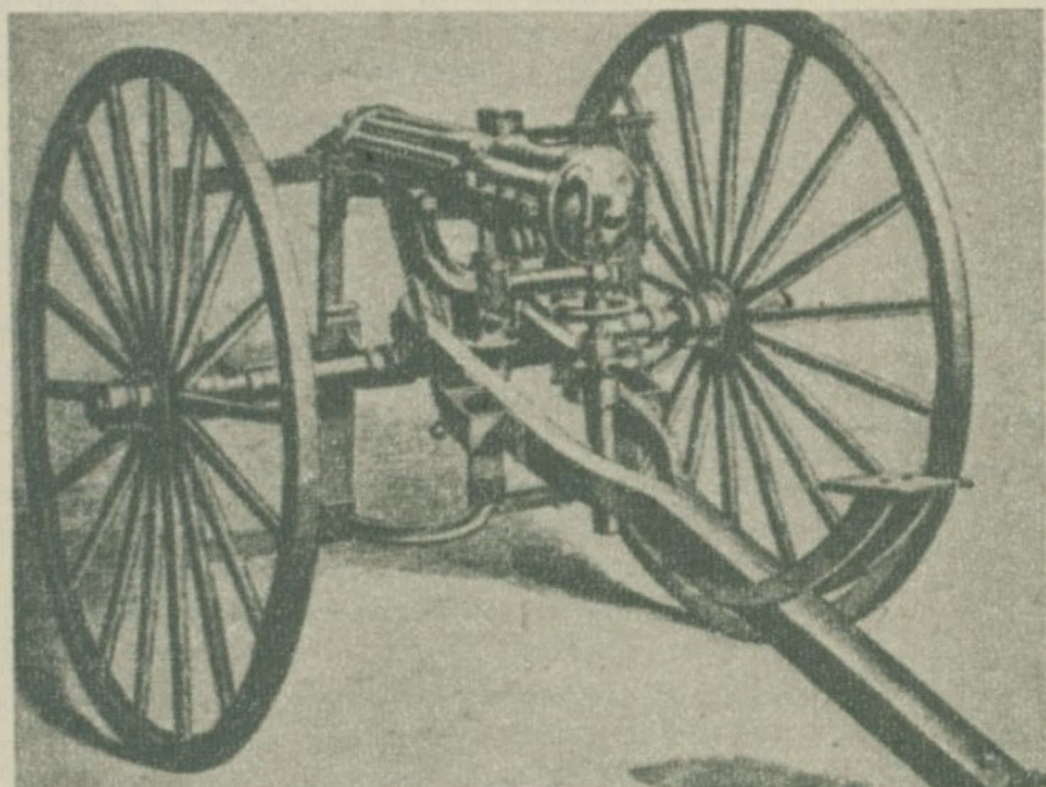
С обзиром да је реч о првом механичком митраљезу, Гетлингов „топ“ био је заиста изузетно брз: 350 метака у минути.
