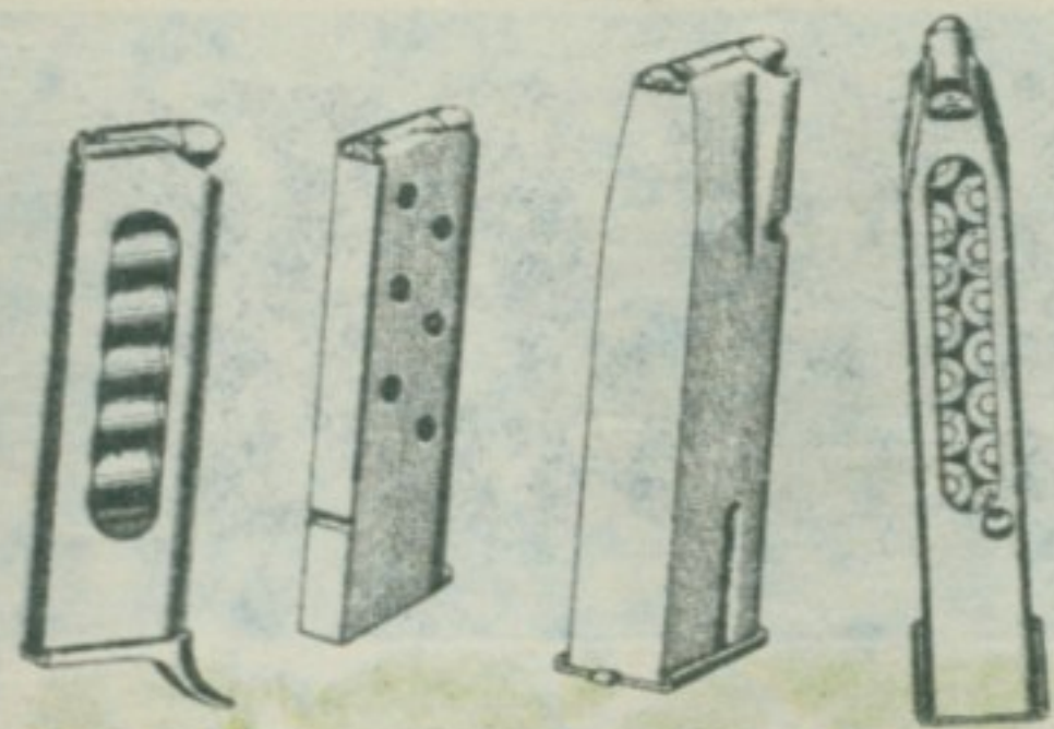
Шаржери за аутоматске пиштоље: Берета М-1934; Браунинг 1900, Браунинг ХП са 13 метака и Берета Ф-92 са 15 метака.
