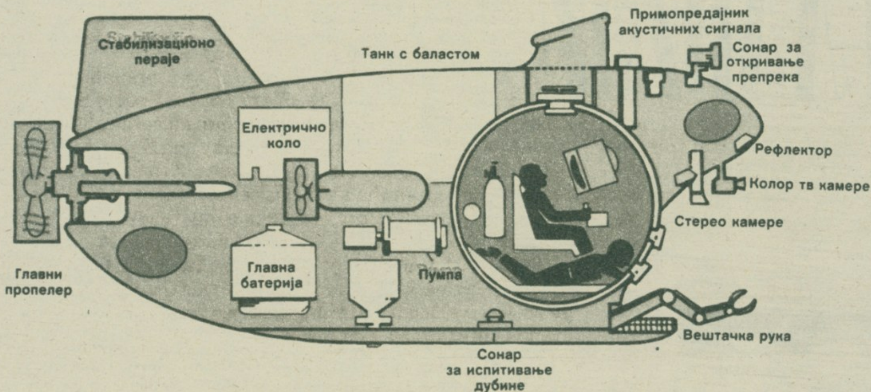
Хиљадама миља под морем: „Шинкаи 6000” имаће облик зрна пасуља, а посада ће бити смештена у кабини од специјалне титанијумске легуре отпорне на притисак.
