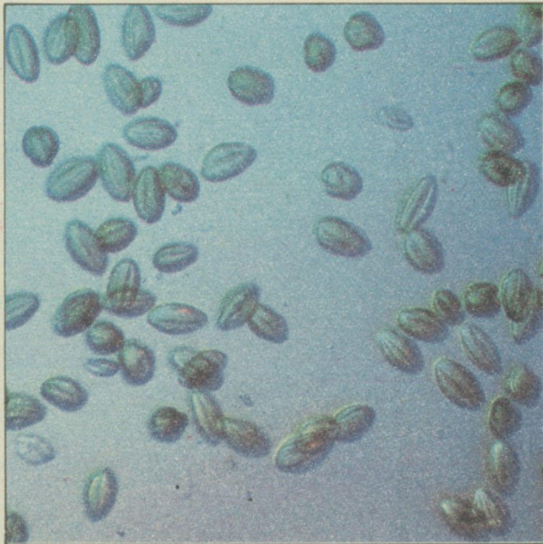
Обична домаћа буђ Полен јаворовог дрвета
