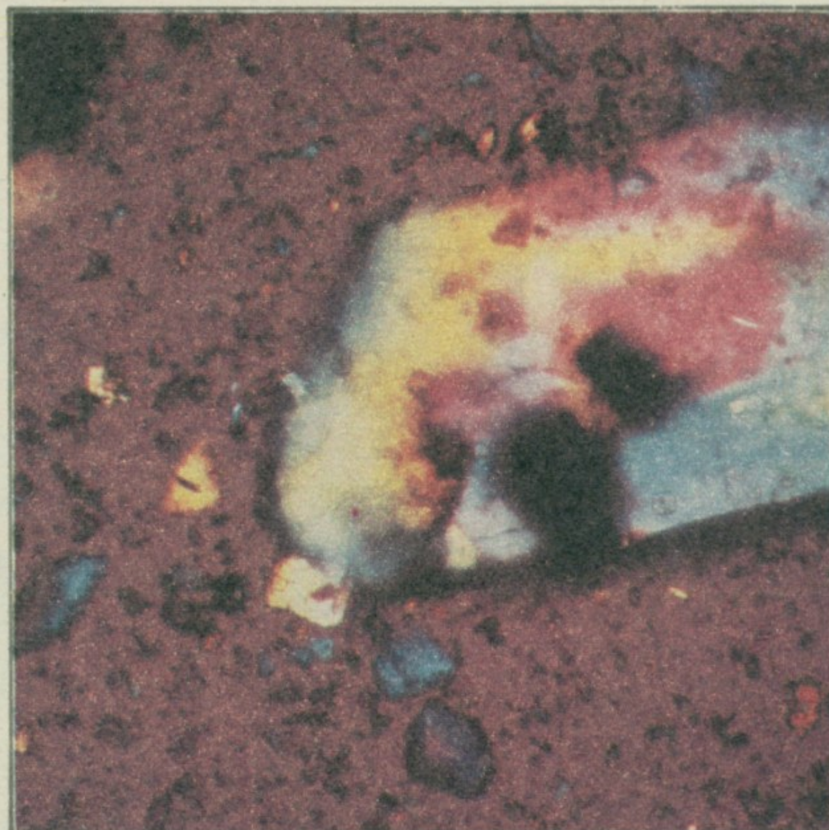
Вулкански пепео са планине Сент Хеленс
