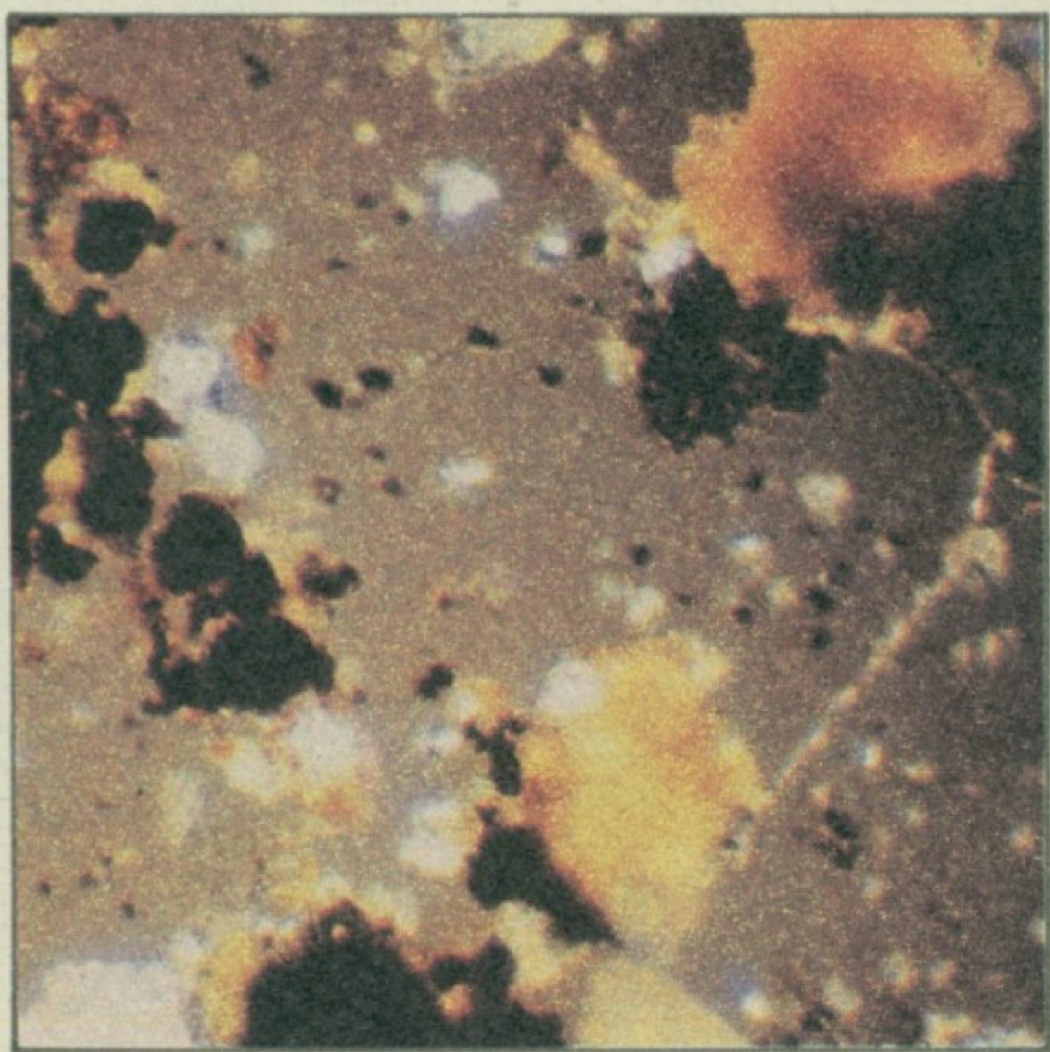
Честице угљеника и сумпора у градском ваздуху
