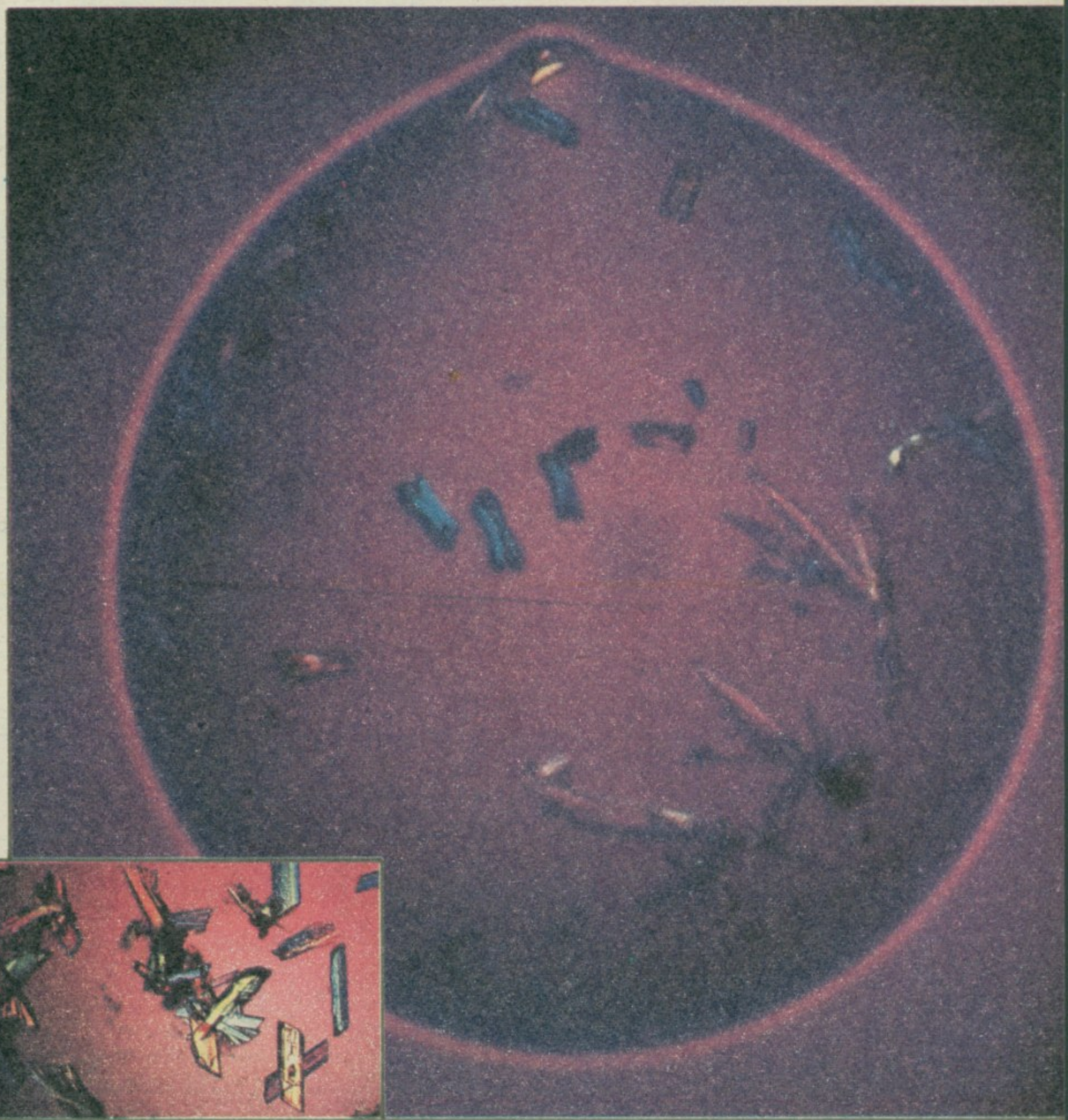
Кап „киселе кише“. Уметнута слика: Игличасти кристали сулфата у једној капљици
