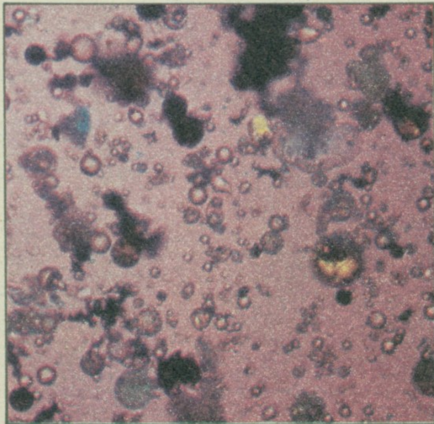
Летећи пепео из термоелектране на угаљ
