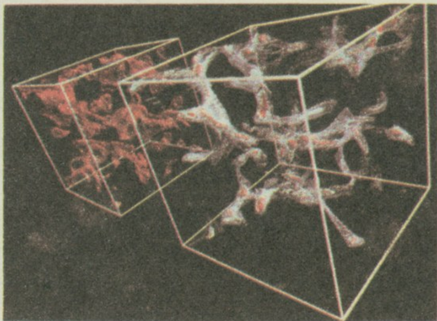
На компјутерској мапи васионе виде се гроздови галаксије
