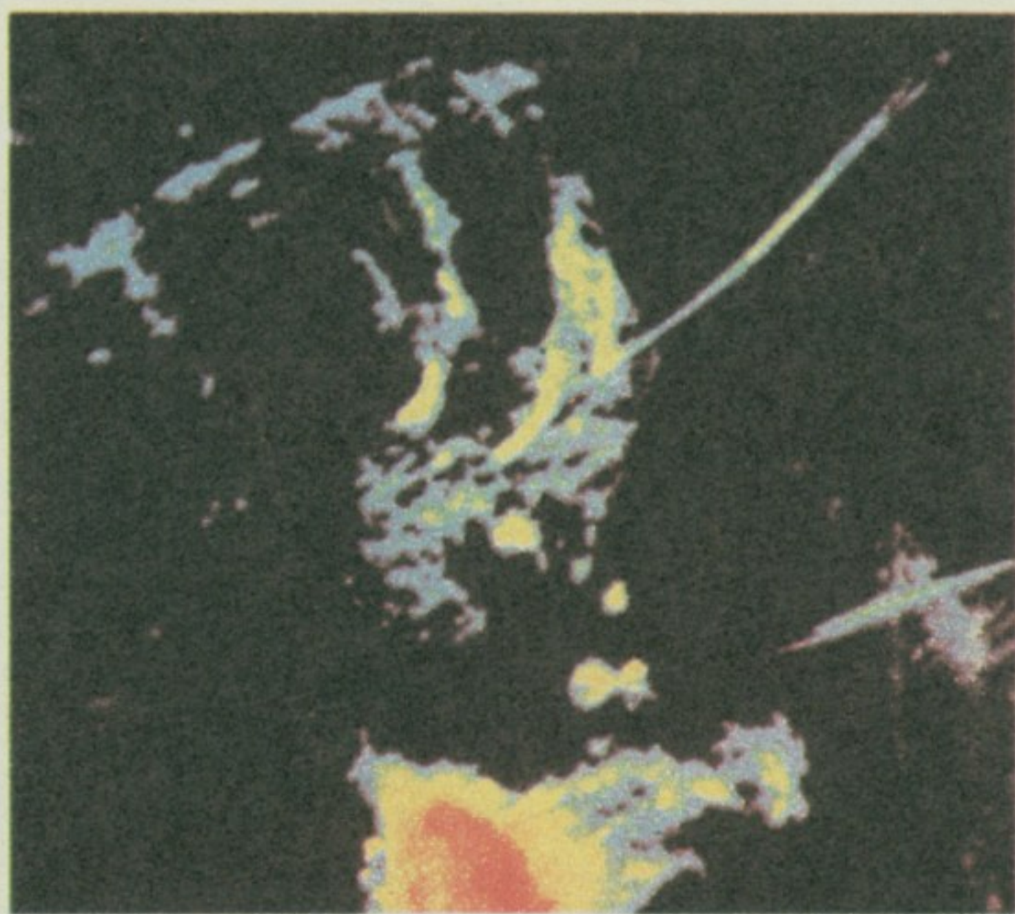
„Влакна“ у средишту Млечног Пута
