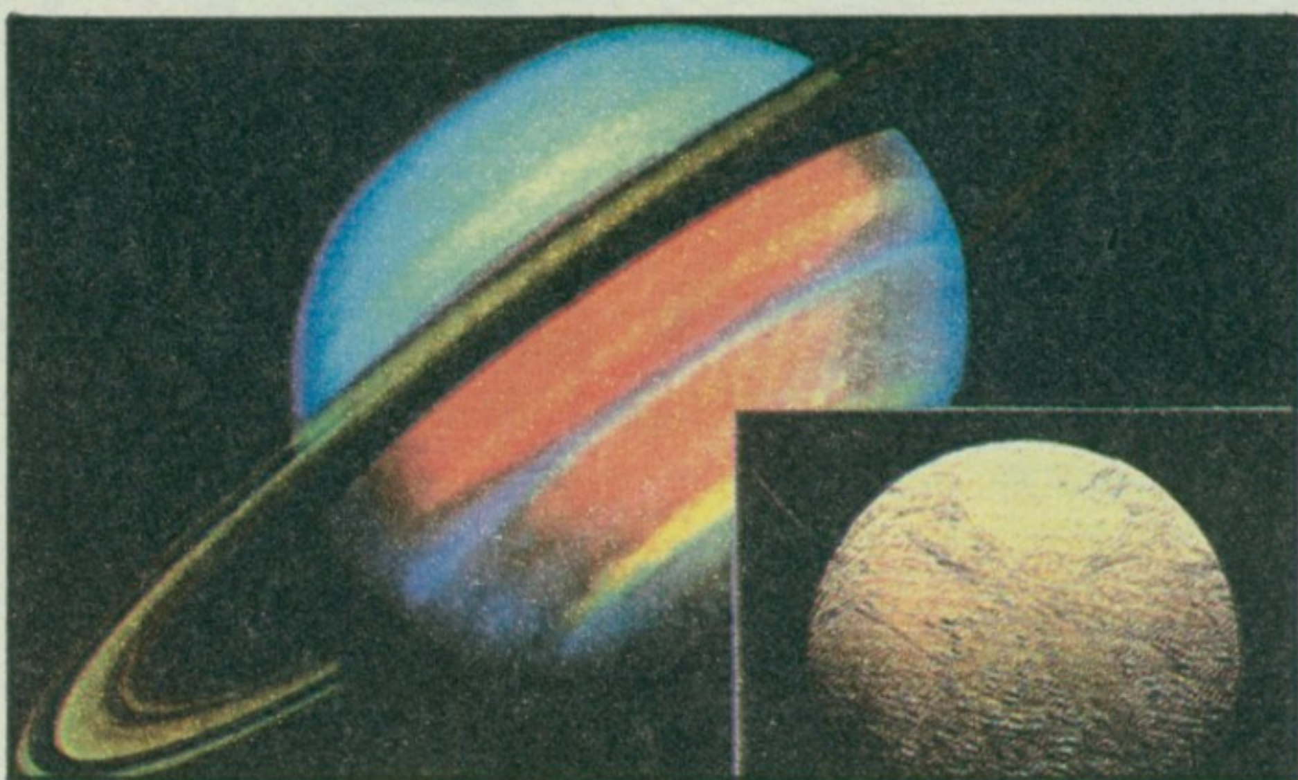
Сатурн у лажним бојама – Појачавањем фотографија „Војаџера“ помоћу различитих боја утврђено је да око ове планете има више слојева атмосфере. Са раздаљине од 118.000 километара „Војаџер“ је такође снимио кратере и удолине на површини једног од преко 15 сателита ове планете.
