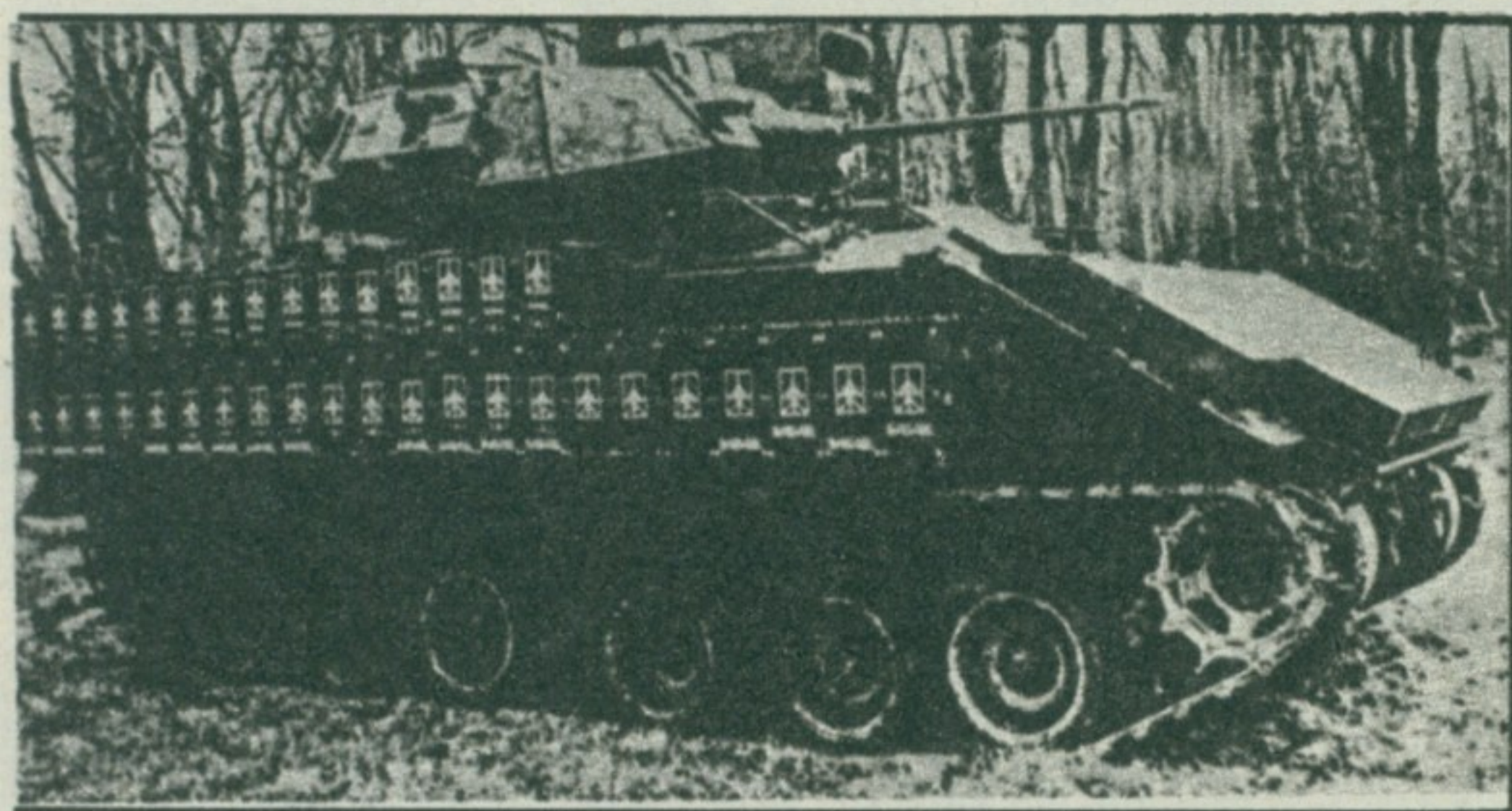
Плоче (кутије) активног оклопа на америчком лаким оклопном возилу „Bradley A2“
