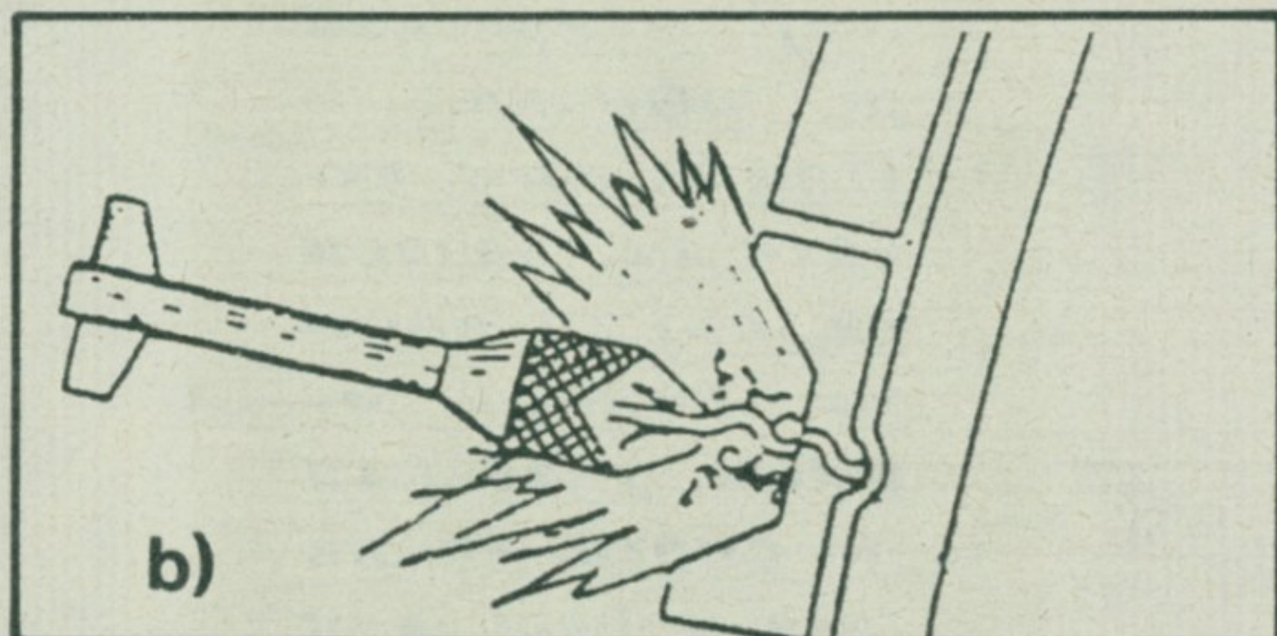
Дејство кумулативног млаза пројектила а) на класичан оклоп, б) на активан оклоп
