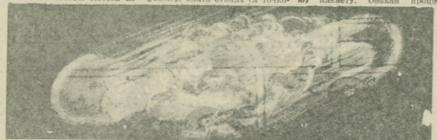
После сусрета неизмерни трилиони врелих гасова претстављали су материју из које су настале планете
