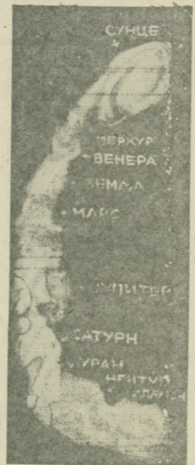
Теорија цигаре: једно огромно испуцале у форми цигаре пролазна Звезда изваукла је из Сунца својом привлачном снагом
