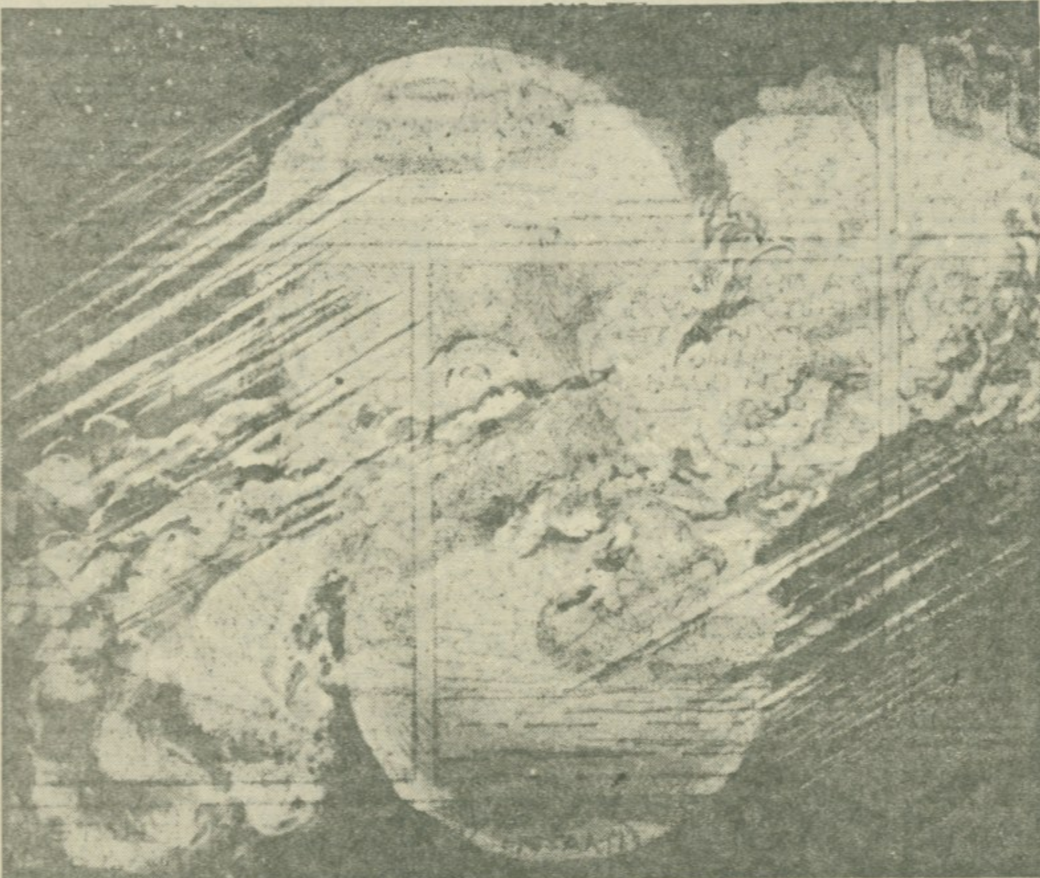
Теорија судара: из „трескотина“ развио се касније сунчани систем.
