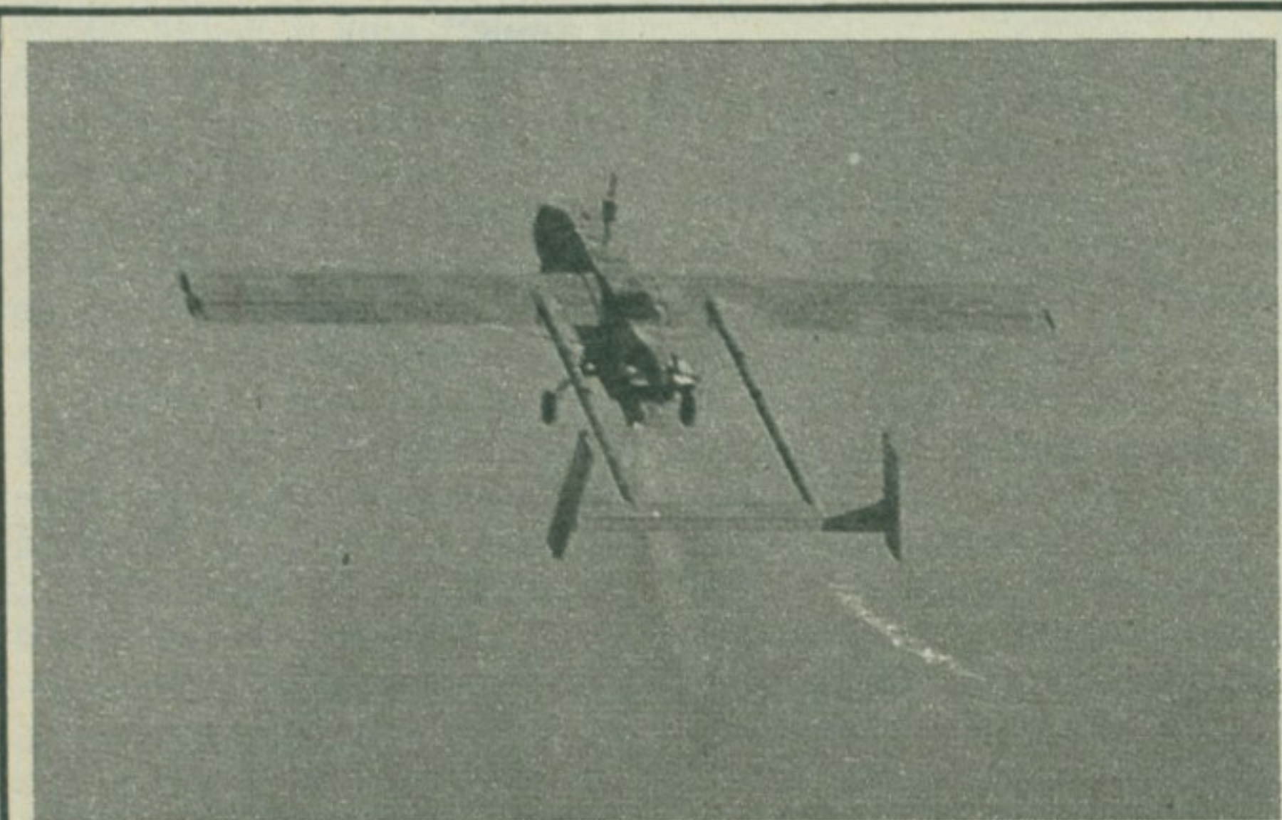
Израелска беспилотна извиђачка летилица „пионир“ полеће
