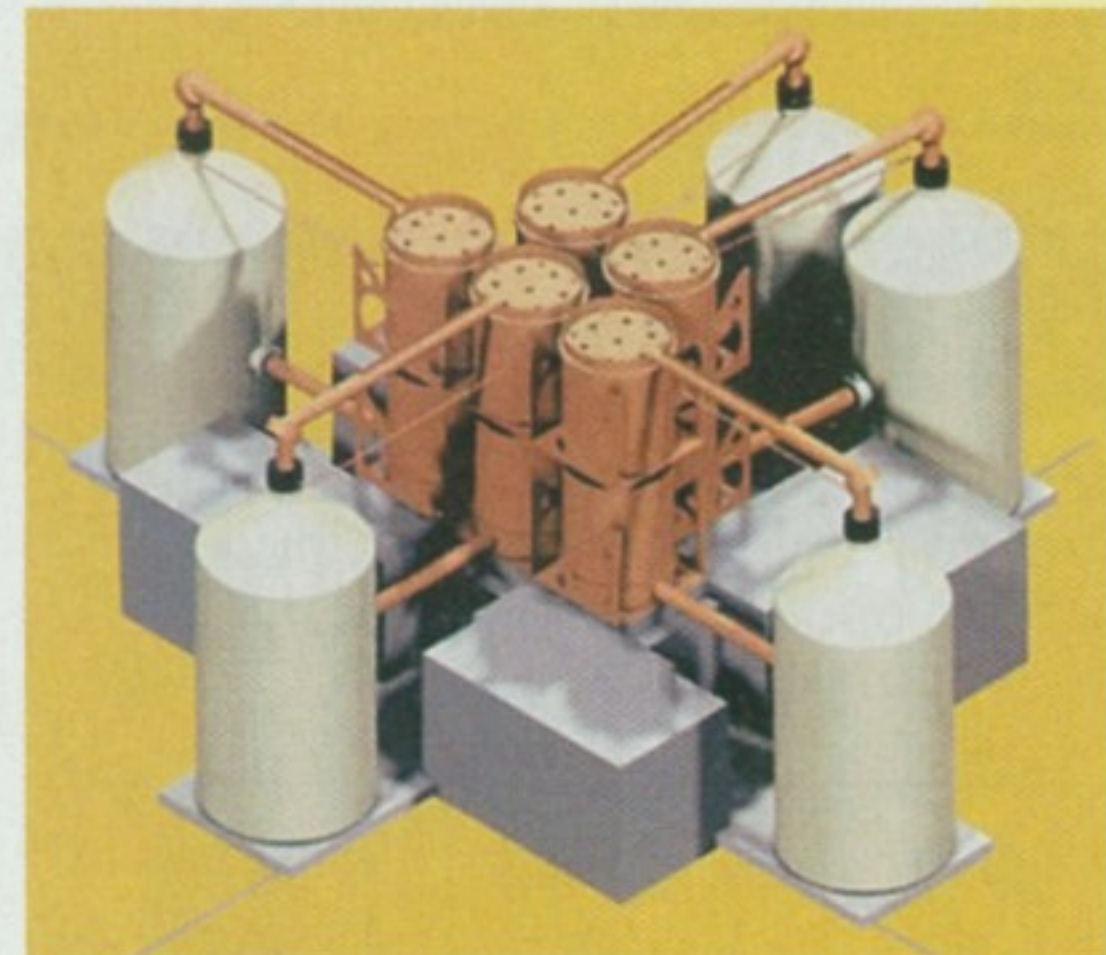
Првеж пројекта „Мајоранин експеримент“, на коме се ради у САД, за проучавање природе неутрина.
